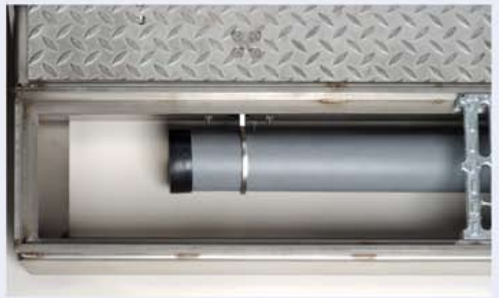
Details zum Schwimmer des MINI Klappschotts
